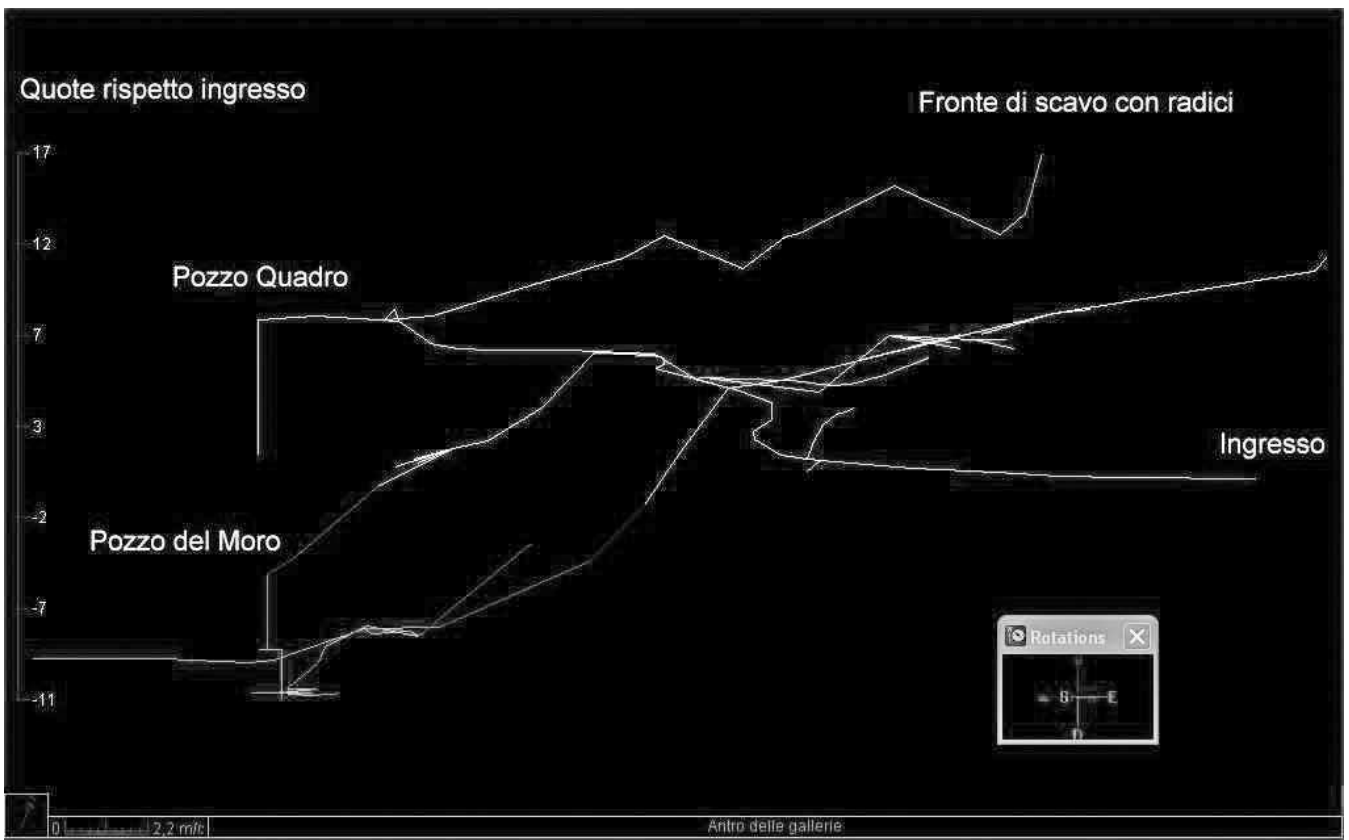
Fig. 11. In alto: rappresentazione tridimensionale della poligonale delle gallerie. In basso: rappresentazione tridimensionale della cavità. Parti rilevate al dicembre 2005. Rappresentazioni eseguite con il software di rilievo speleologico Compass.
